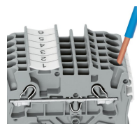
Raccordement du conducteur – insertion directe.
