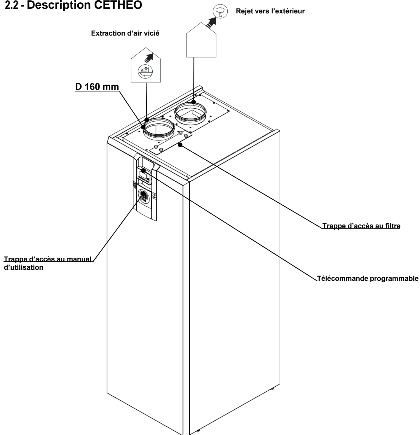
Fig. 4: Description composants principaux CETHEO
