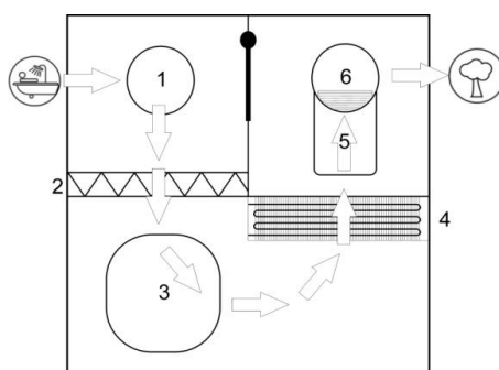
Fig. 3: Fonctionnement Ventilation + PAC
