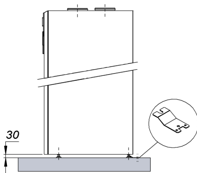
Fig. 6 : Permet le passage de l'alimentation Eau Froide et départ Eau Chaude. Fixer le CETHEO au sol à l'aide d'une des pattes de transport.
