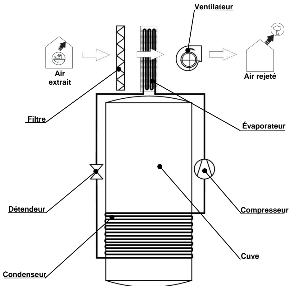
Fig. 1: Principe de fonctionnement CETHEO
