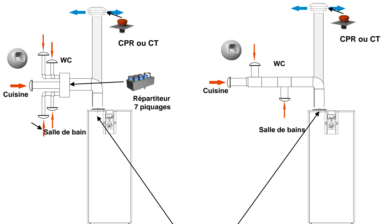
Fig. 8: Exemple de montage par "Répartition"
