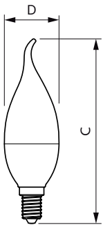
MASTER LEDcandle DT 5.5-40W E14 BA38 CL
