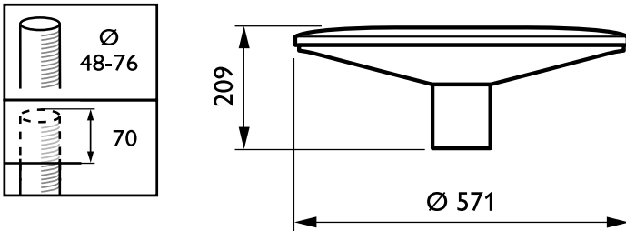
BDP100 LED50/730 II DS PCC GR 62P
