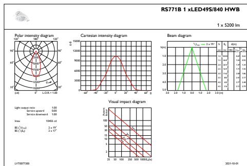
IFAS1_RS771B1xLED49S840HWB
