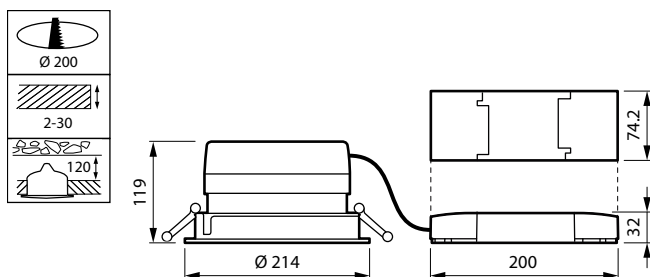
DN571B LED12S/840 DIA-VLC-E C WH
