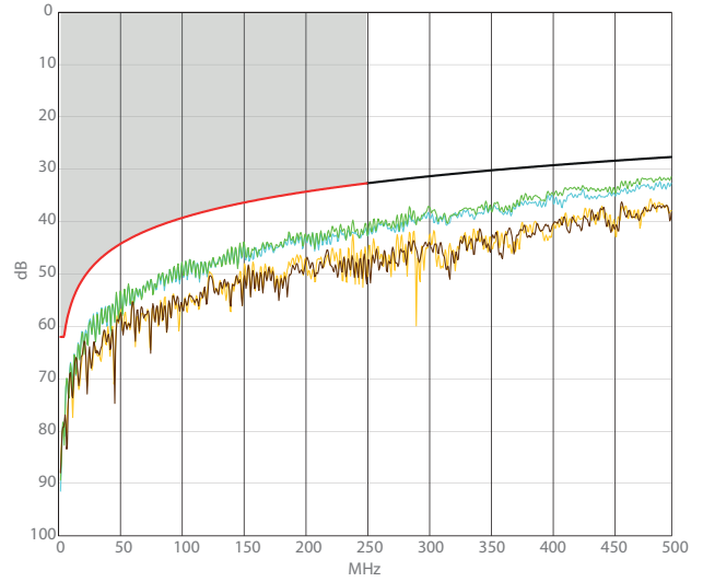
ACR (Atténuation to Crosstalk Ratio) (Ecart paradiaphonique)
