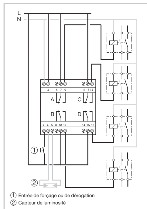
Image 3 : schéma de raccordement EGN400 (4 sorties)
