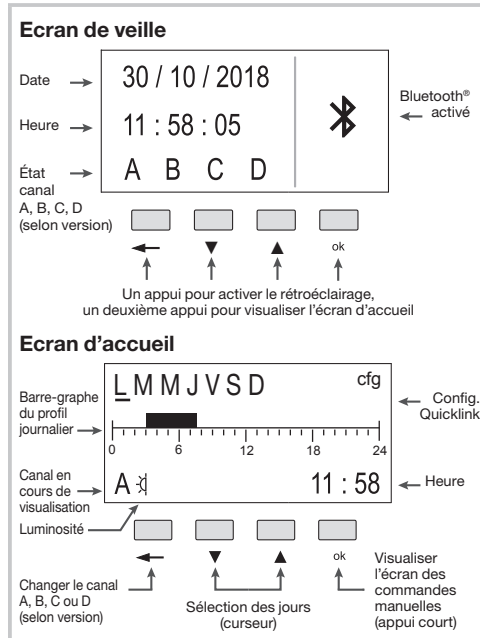
Image 1 : présentation de l'écran de veille et d'accueil
