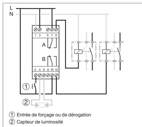
Image 2 : schéma de raccordement EGN200 (2 sorties)
