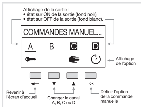
Image 4 : présentation de l'écran des commandes manuelles.
