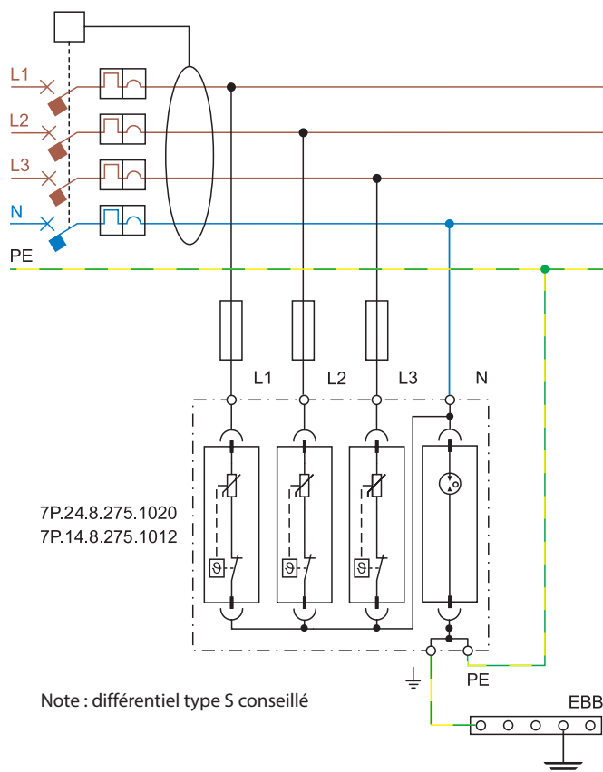
TT ou TN-S TRIPHASÉ EN AVANT DU DIFFÉRENTIEL
