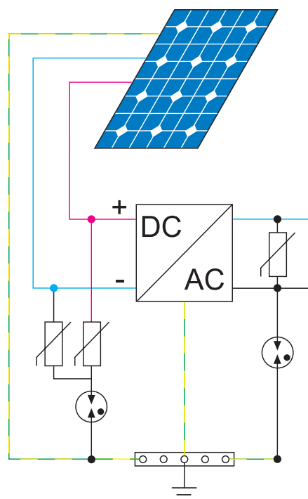
Figure 10 : schéma d'une installation photovoltaïque sur un bâtiment sans paratonnerre, protégée sur le coté DC par un parafoudre avec U_{OCSTC} = 420 \text{ V} , et sur le coté AC par un 7P.22 spécifique pour installation schéma TT.
