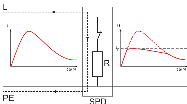
Figure 4 : limitation des surtensions
