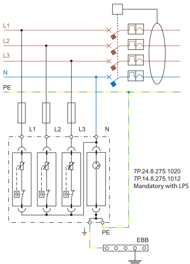
TT TRIPHASÉ EN AMONT DU DIFFÉRENTIEL
