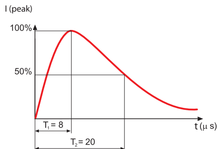
Figure 6 : forme d'onde de courant 8/20μs
