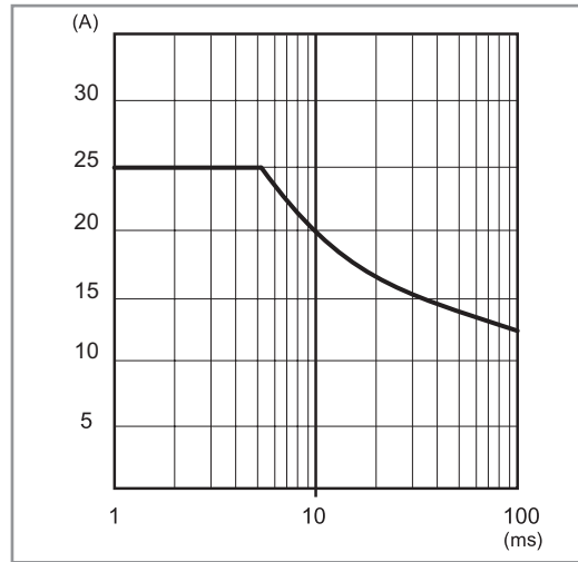
P78-10 Pic de courant en sortie en fonction du temps(78.2A)
