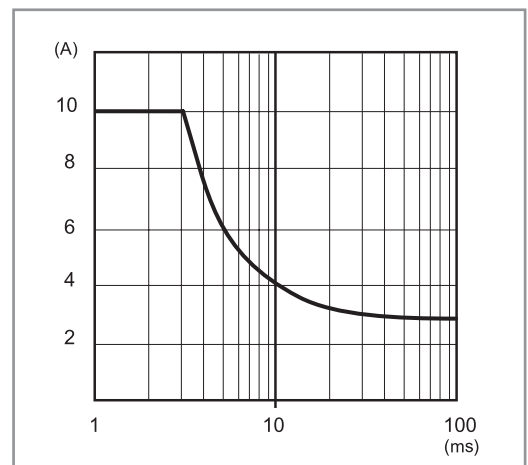
P78-4 Pic de courant en sortie en fonction du temps (78.60)
