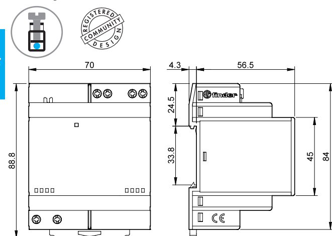
Type 78.36 Bornes à cage
