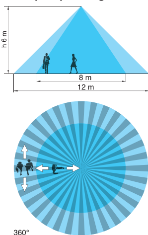
18.31...0031 - Montage en saillie ou encastré pour plafond grande hauteur
