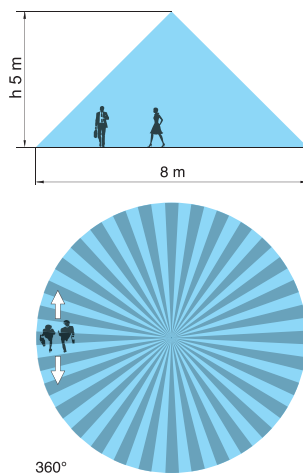
18.21.8.230.0000 - Montage en saillie 18.31.8.230.0000 - Montage encastré
