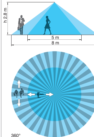
18.31...0031 - Montage en saillie ou montage encastré
