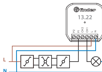
Installation connectée
