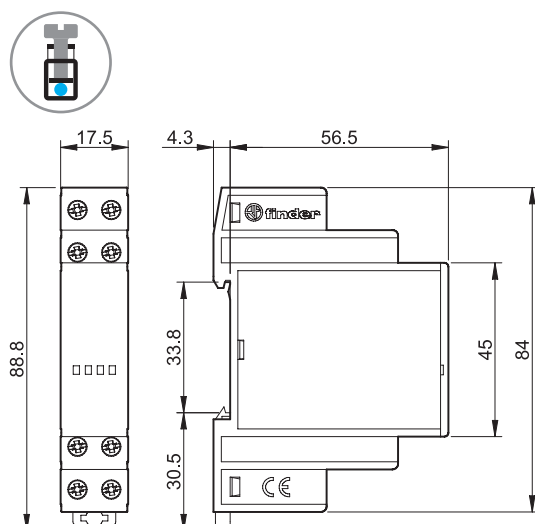
13.12 Bornes à cage
