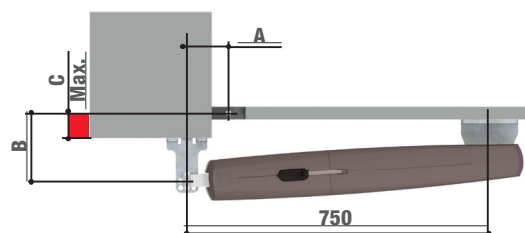
MOTEUR DROIT VU DE L'INTÉRIEUR
