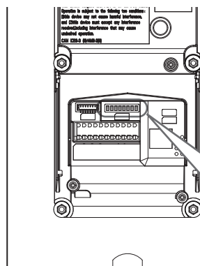
Commutateurs DIP
