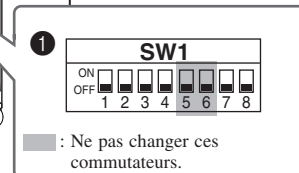
Commutateurs DIP
