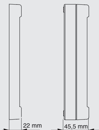
Encastrement
