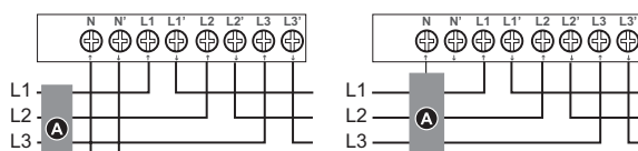
3PH4W
