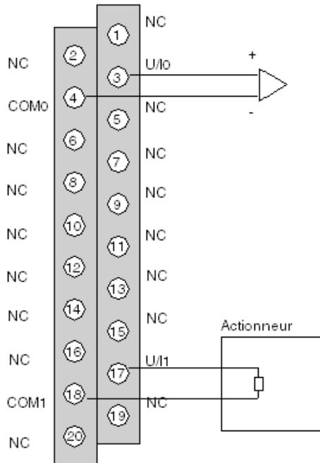
Vue côté câblage
