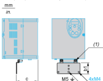
(1) 2 vis M5
