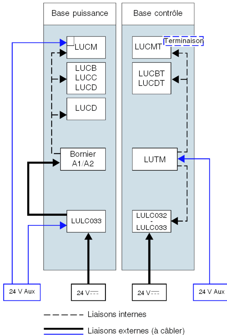
Schéma des alimentations 24 V \overline{\text{---}} et 24 V aux
