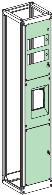
Compact NS 630/1600 3P/4P Masterpact NT 630/1600 3P
