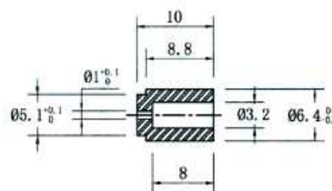
Bague plastique
