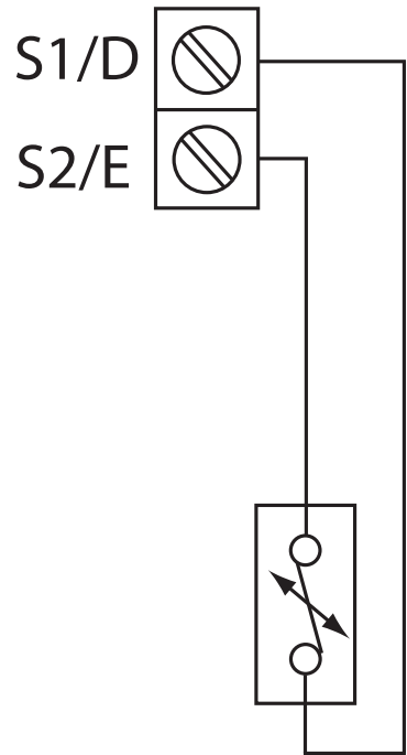
Configuration pour capteur d'ambiance à distance ou pour capteur de limite
