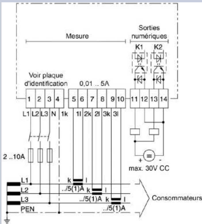
UMG 96L / UMG 96
