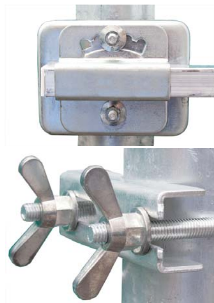
Bride renforcée avec écrous papillons moulés sous pression
