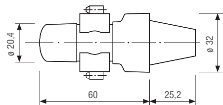
Montage apparent sonde LF
