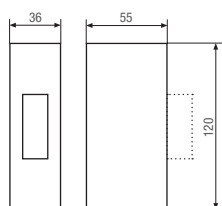
Kit montage en saillie 1 UM
