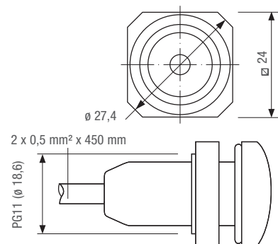
Montage encastré sonde LF
