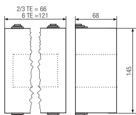
Kit montage en saillie 2, 3, 6 UM
