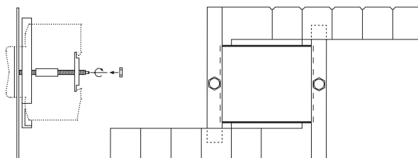
Panneau d'encastement mural 1-6 UM
