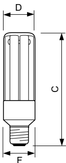
PL E-R Polar 23W/827 E27 220-240V
